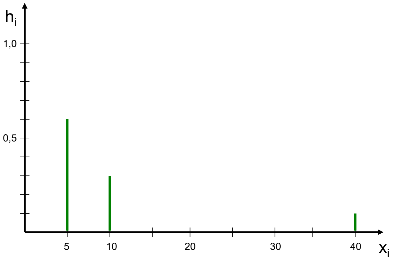
Abb. 15b: Verteilungsfunktion 1
