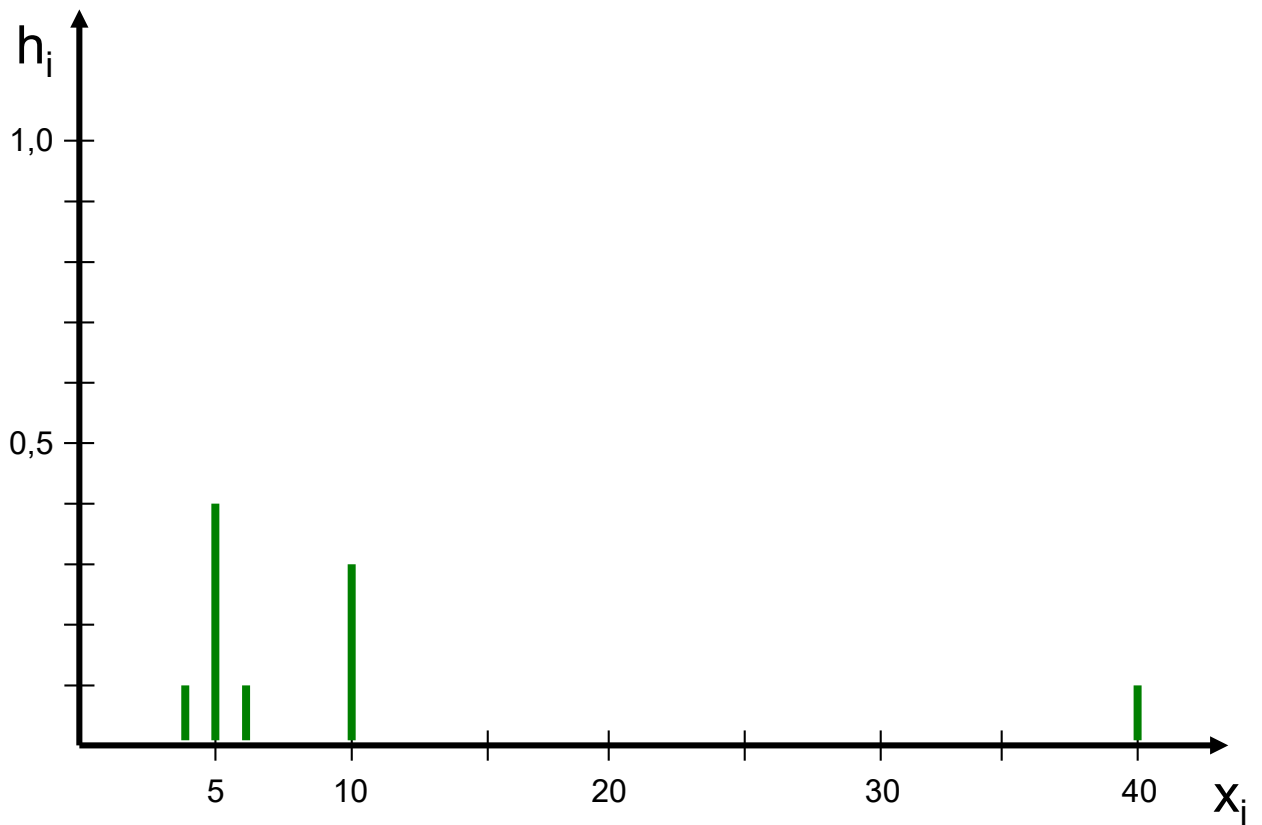
Abb. 16b: Verteilungsfunktion 2
